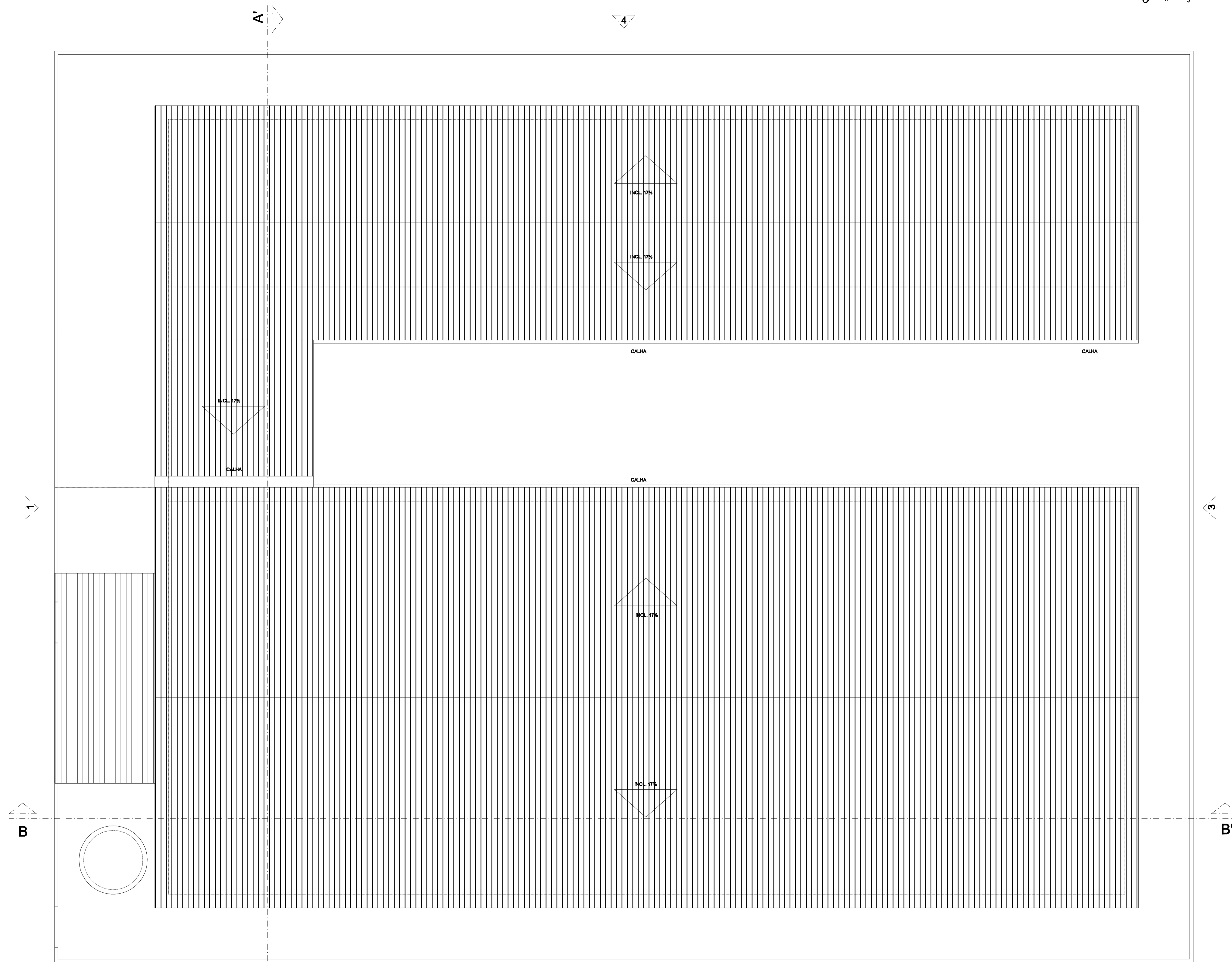
PLANTA COBERTURA ESCALA 1:100
